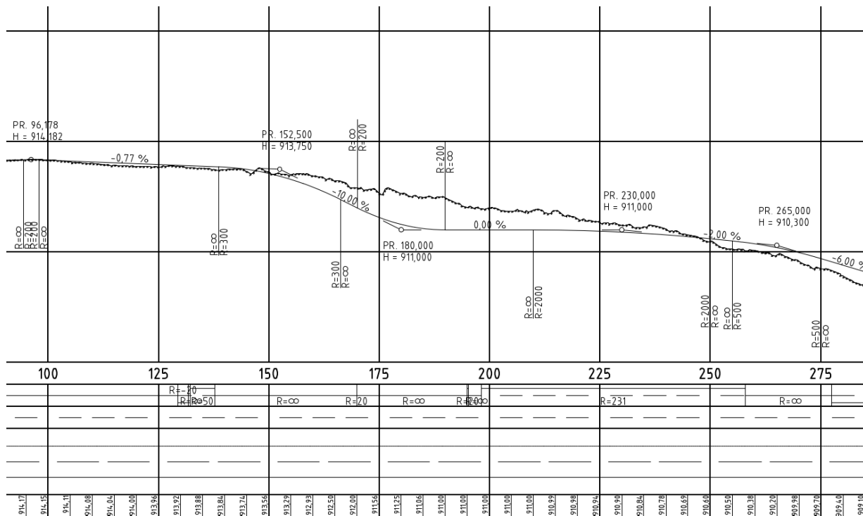
Figur 59: Utsnitt av lengdeprofil for KV5 - Lokkarstigen. Vegen senkes ca. 2 meter inn mot krysset ved Syvervegen.
