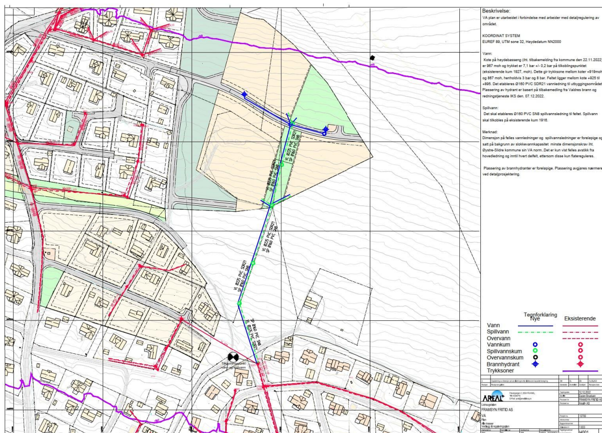
Figur 38: Overordnet VA-plan.
