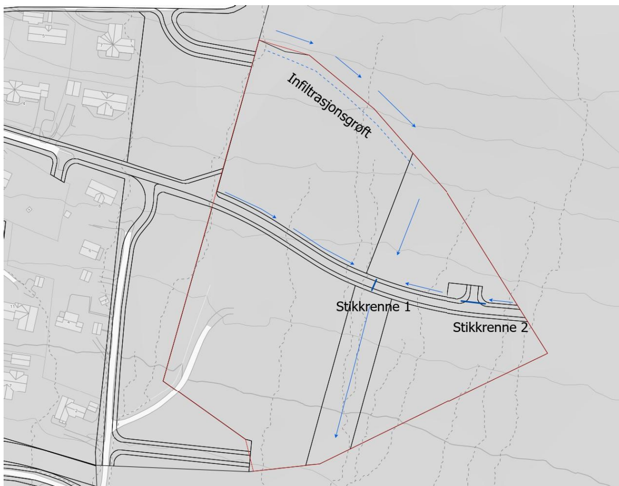
Figur 40: Overvannsplan.
