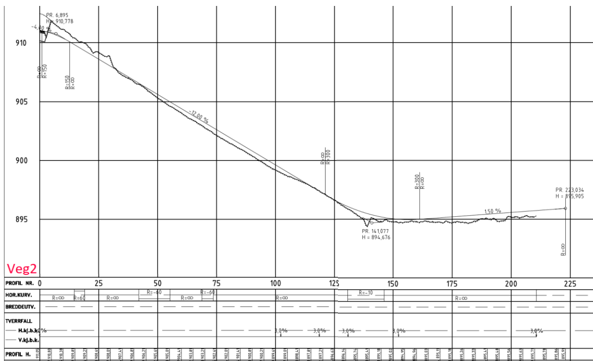
Figur 58: Lengdeprofil for KV6 - Syvervegen.
